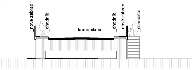
ŘEZ C-C'
