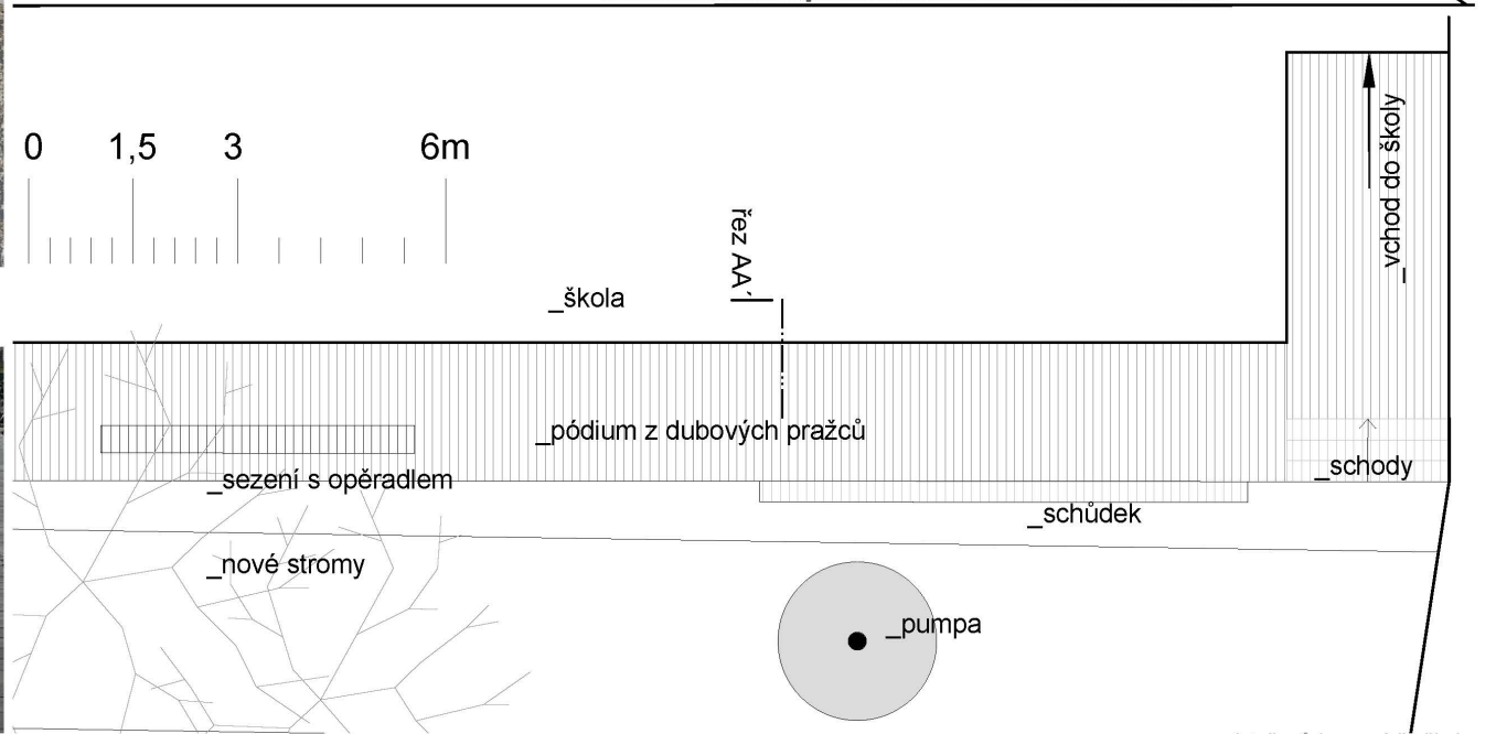
detail, půdorys pódia školy
