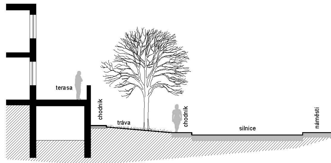
řez BB
