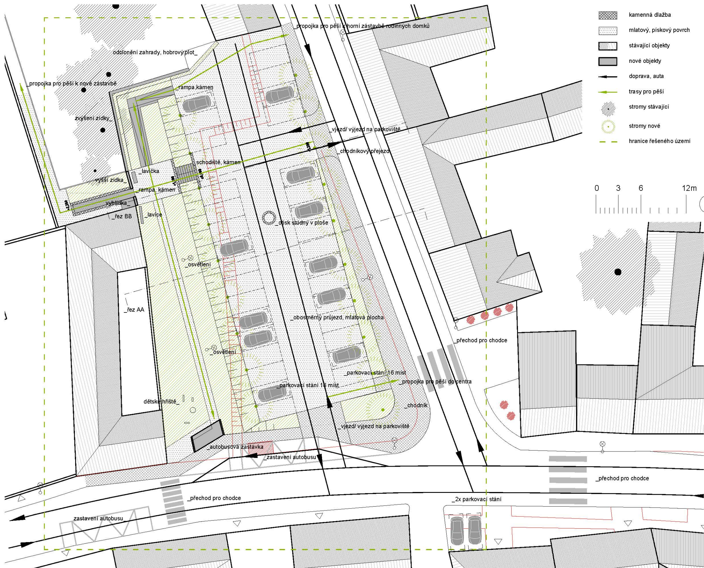
Nové horní parkoviště, situace
