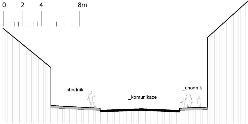
ŘEZ B-B'
